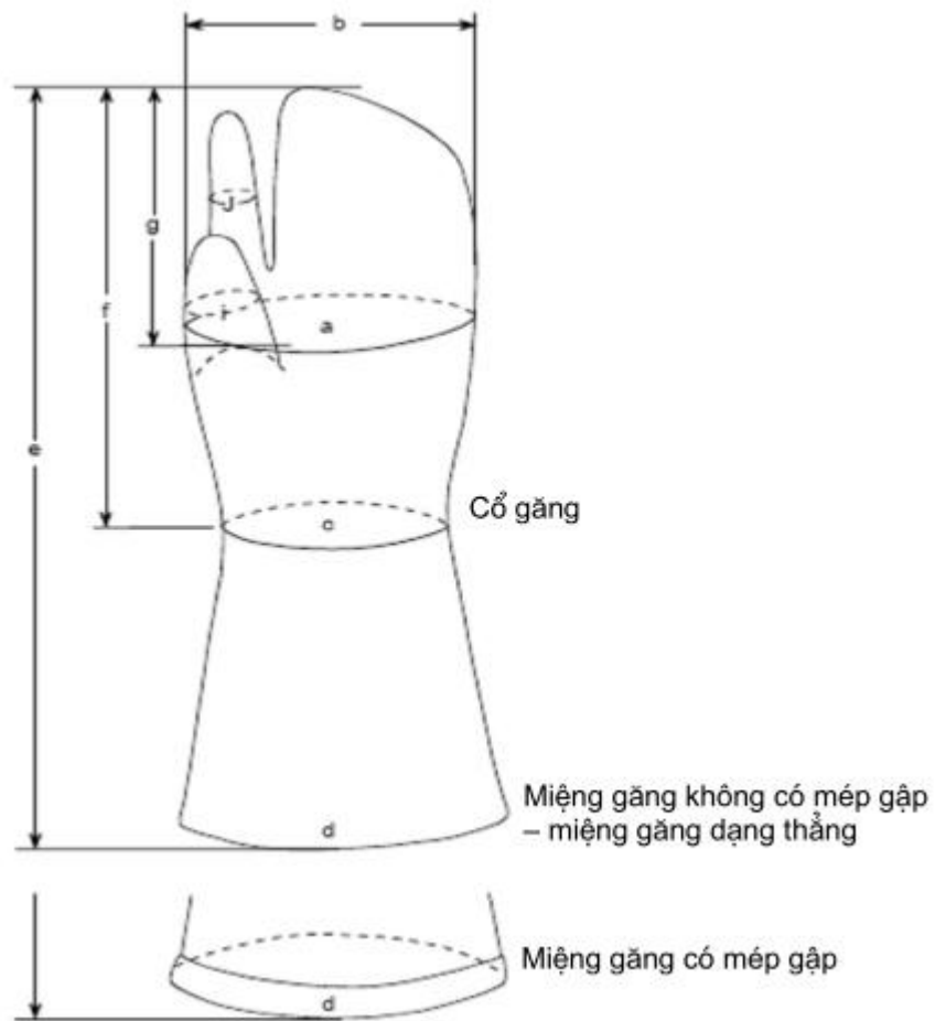
Hình 2 – Hình dạng găng tay bao nhiều ngón
