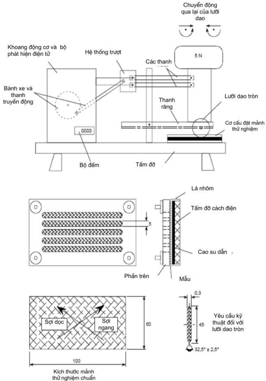
Hình 13 – Trang bị để thử nghiệm khả năng chịu cắt (xem 9.2)
