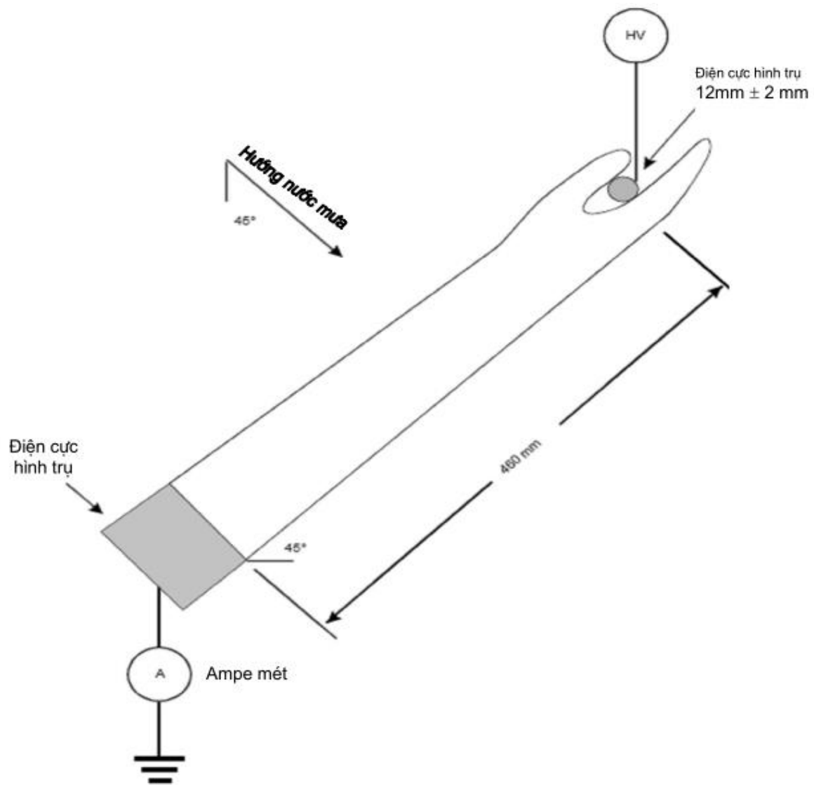
Hình 16 – Bố trí để thử nghiệm dòng điện rò (xem 10.2)
