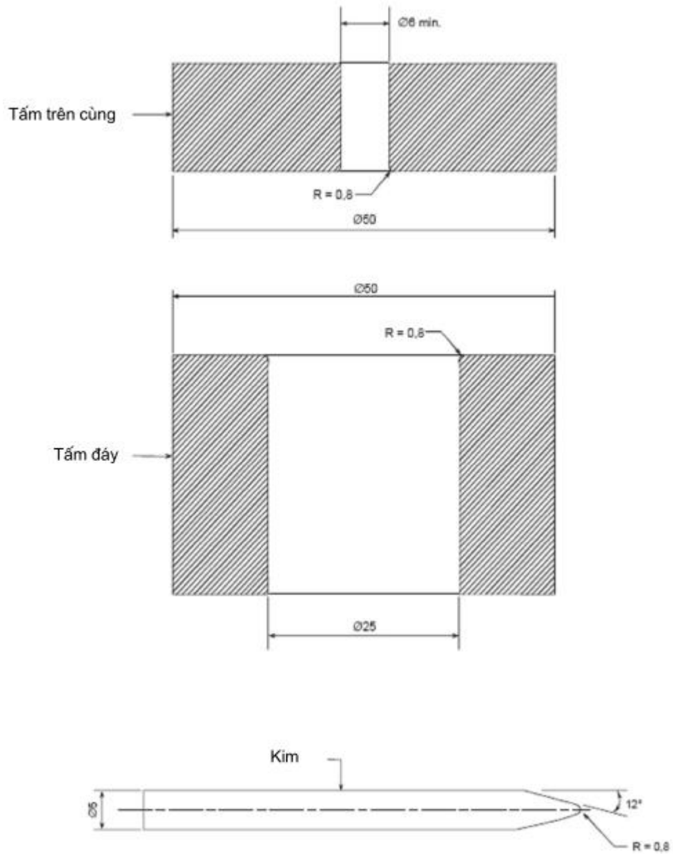
Hình 7 – Tấm thử nghiệm và kim dùng cho thử nghiệm khả năng chịu xuyên thủng về cơ (xem 8.3.2)
