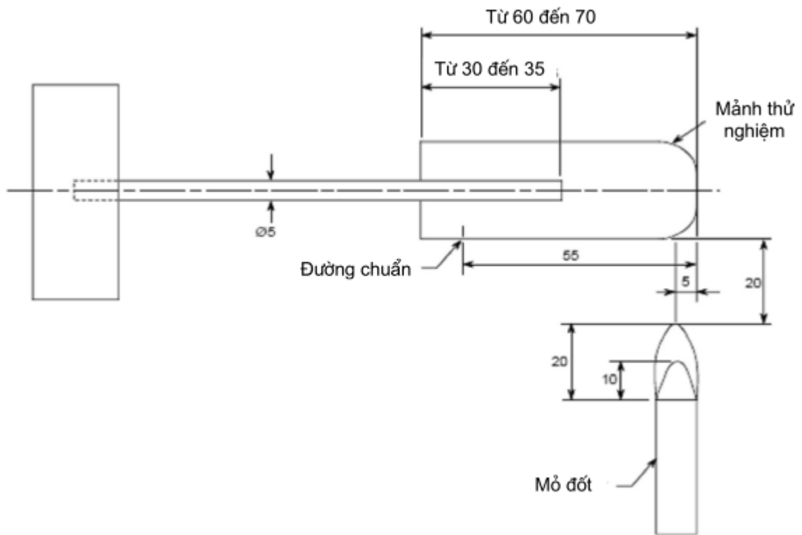
Hình 11 – Bố trí dùng cho thử nghiệm chày chày (xem 8.6.2)
