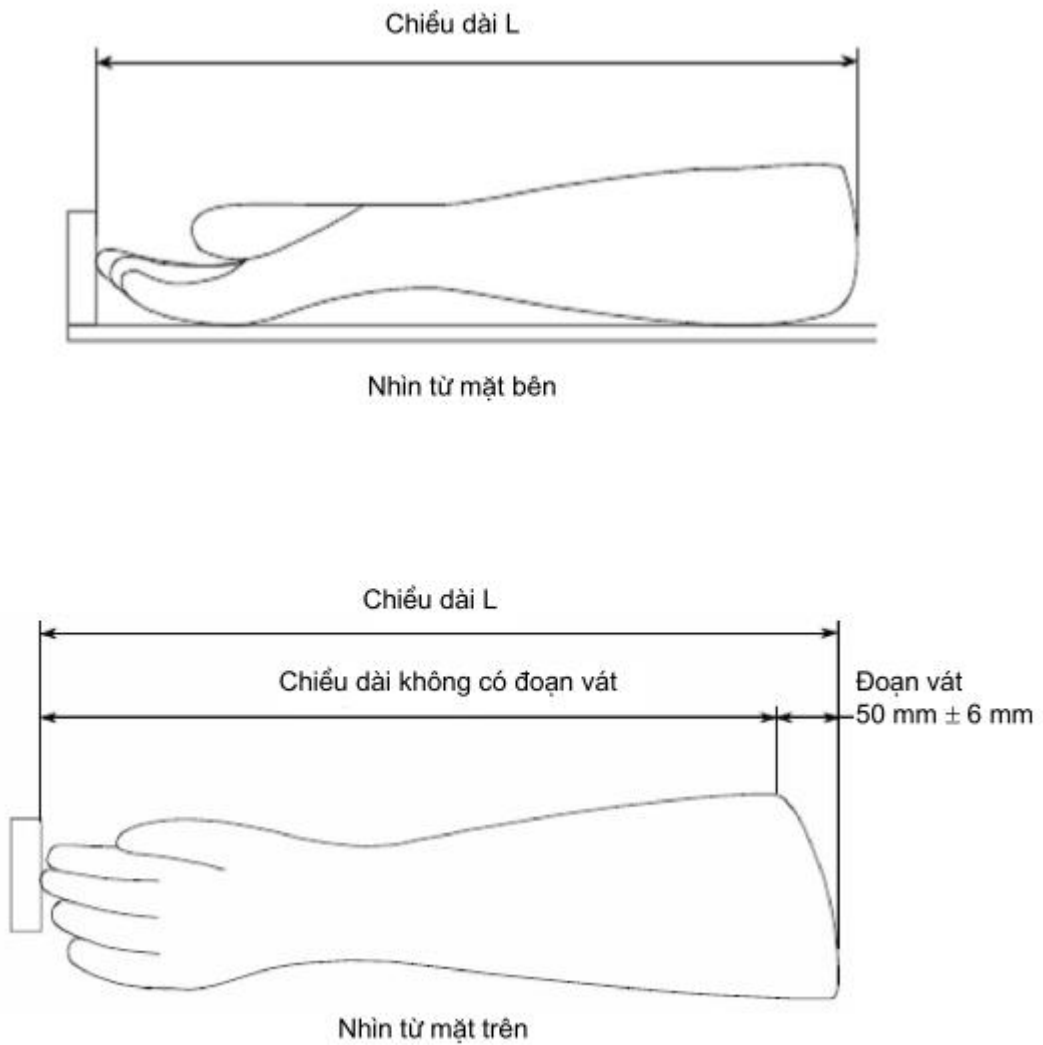
Hình 3 – Đoạn vát của găng tay (xem 8.2.2)
