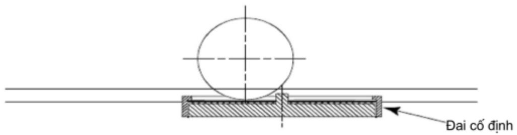
Hình 12a – Nhìn theo A-A
