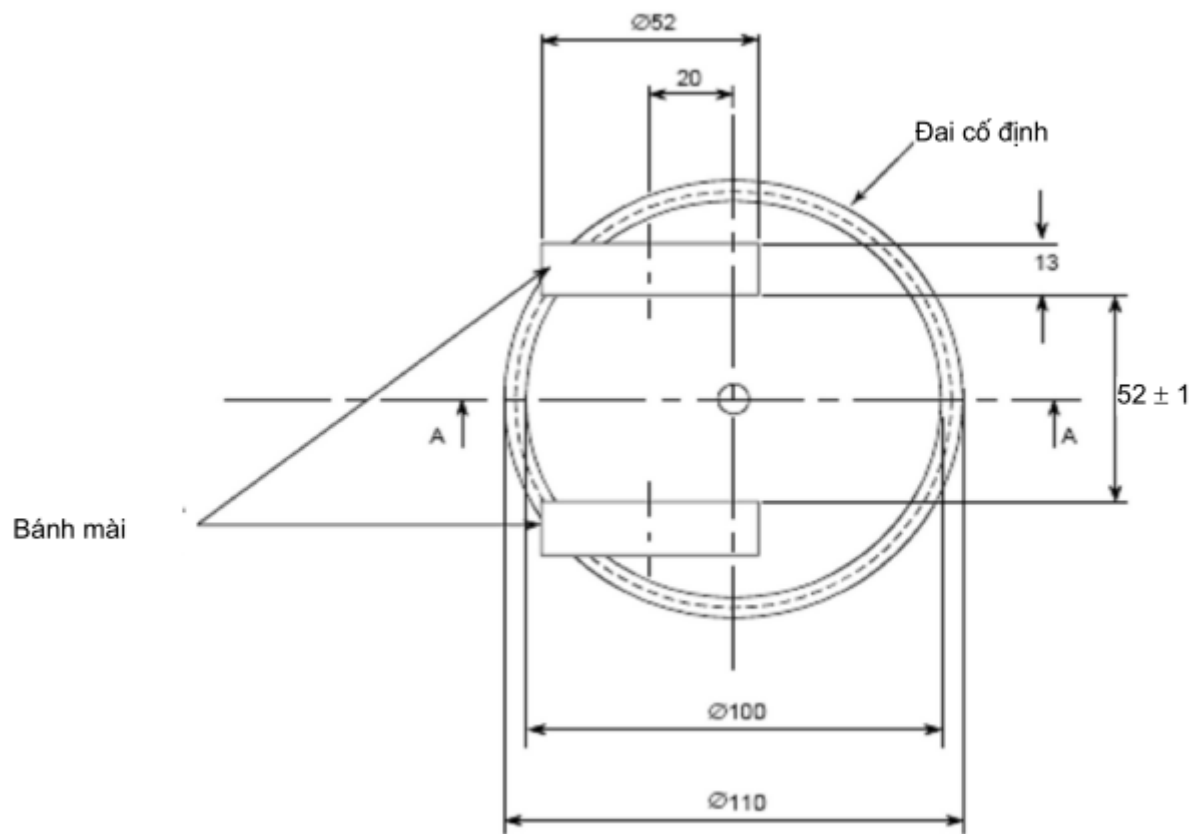
Hình 12b – Nhìn từ trên xuống
