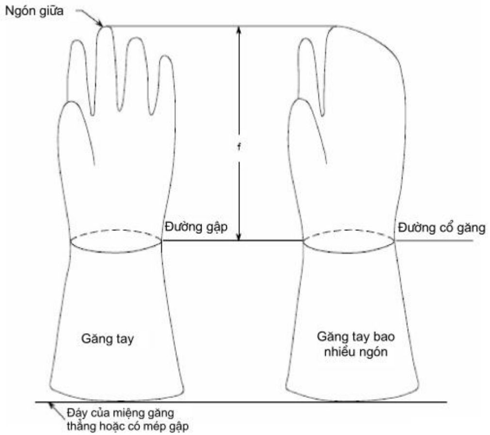
Hình 9 – Đường uốn (gập) dùng cho thử nghiệm nhiệt độ cực thấp (xem 8.6.1 và 8.7.4)
