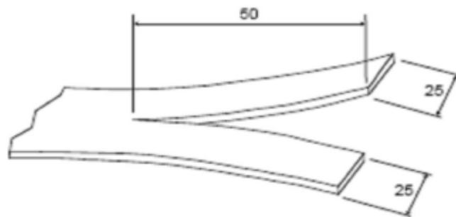
Hình 15 – Hình dạng mảnh thử nghiệm để thử nghiệm khả năng chịu xé (xem 9.3)
