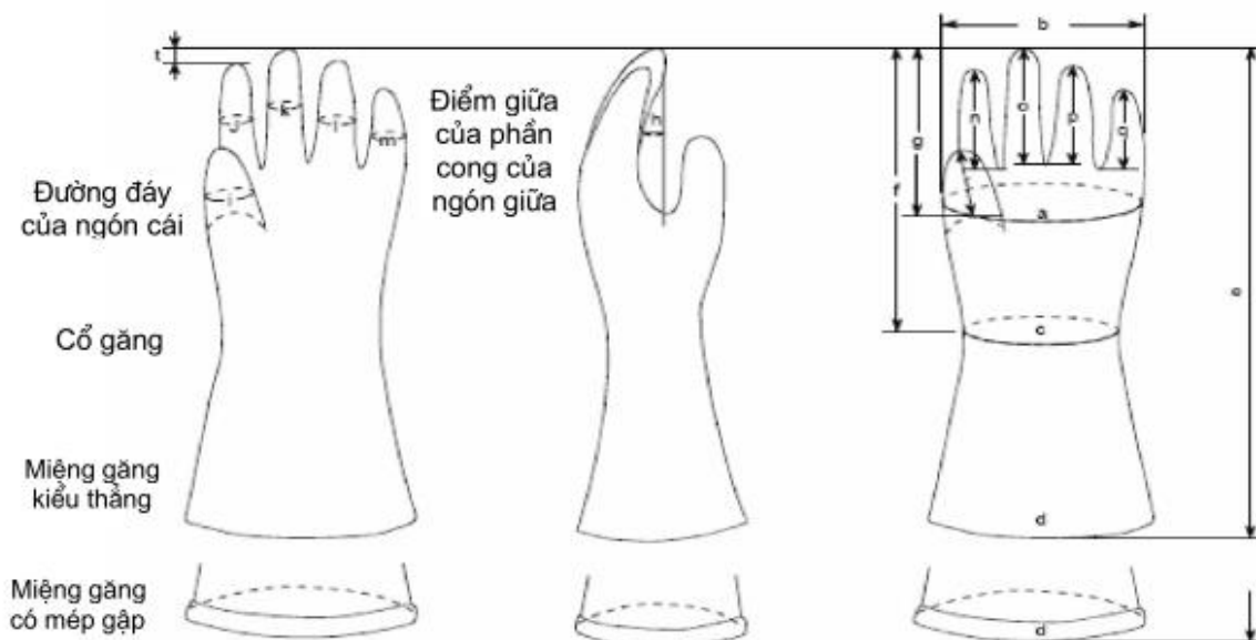
Hình 1a – Hình dạng của găng tay
