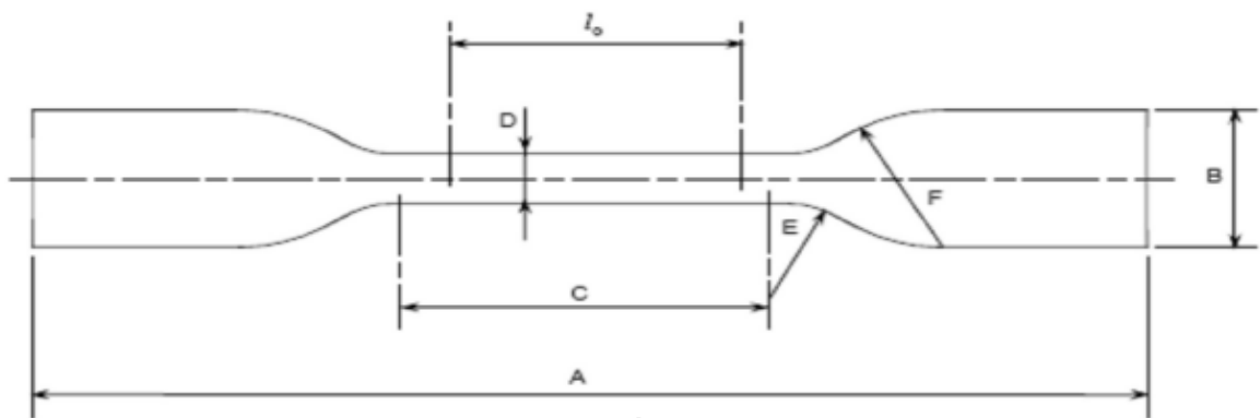
Hình chiếu bằng
