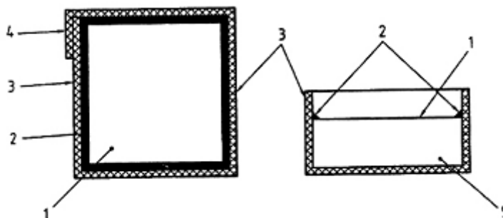
Hình B.1 - Mặt cắt ngang của mẫu bọc tấm cao su và vết gắn keo (bên phải) và nhìn mẫu từ trên (bên trái)
