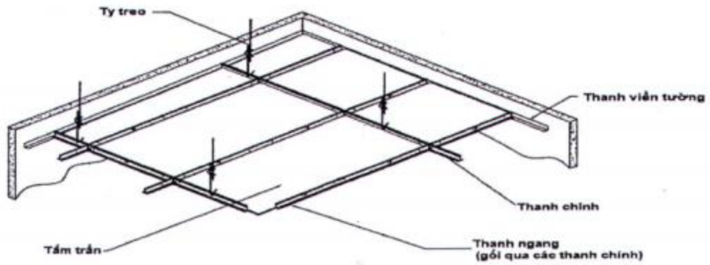
a. Hệ trần treo trực tiếp
