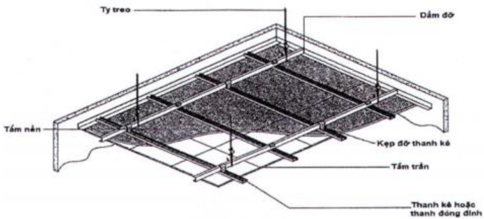
c. Hệ trần treo thanh lót
