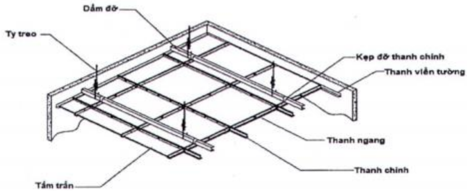
b. Hệ trần treo gián tiếp
