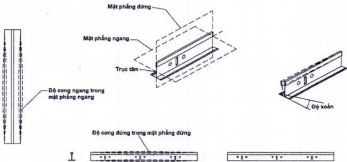
Hình 2 - Hình vẽ thể hiện độ cong ngang, độ cong đứng và độ xoắn
